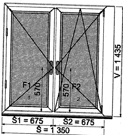
Konštrukcia otváracia dovnútra - pohľad zvnútra
